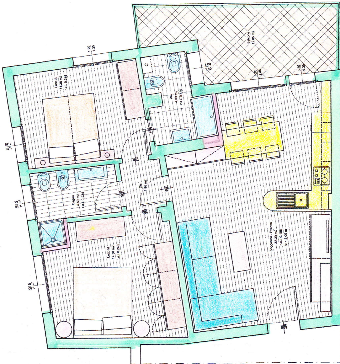
PIANTA PIANO TERZO SCALA 1 : 50
